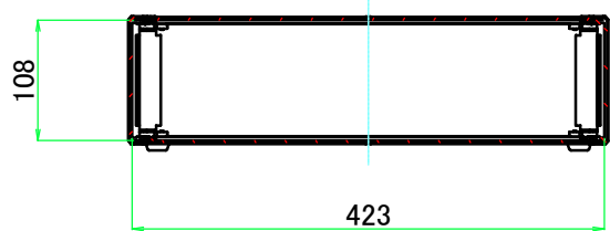
B-B ( 1 : 7.5 )
