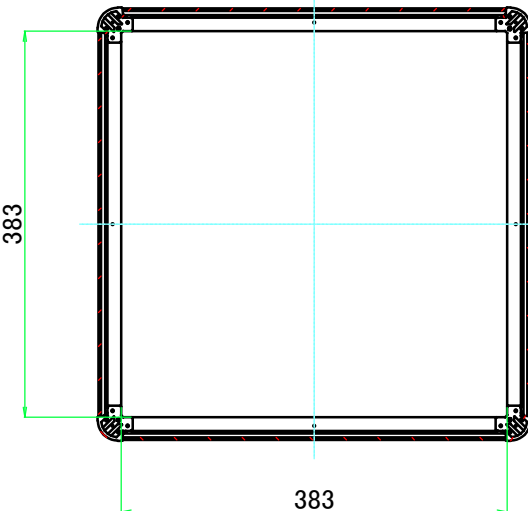
C-C ( 1 : 7.5 )
