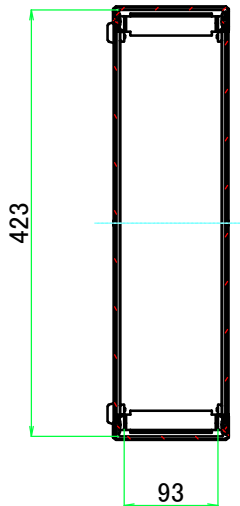
A-A ( 1 : 7.5 )
