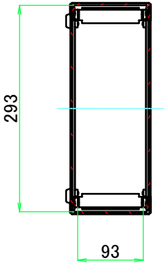
A-A ( 1 : 7.5 )
