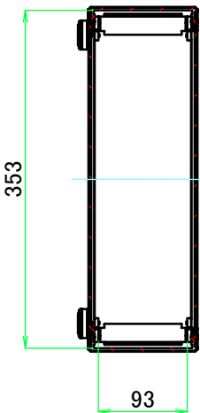
A-A (1:7)
