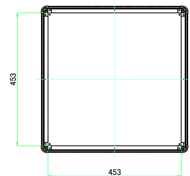
C-C ( 1 : 8 )
