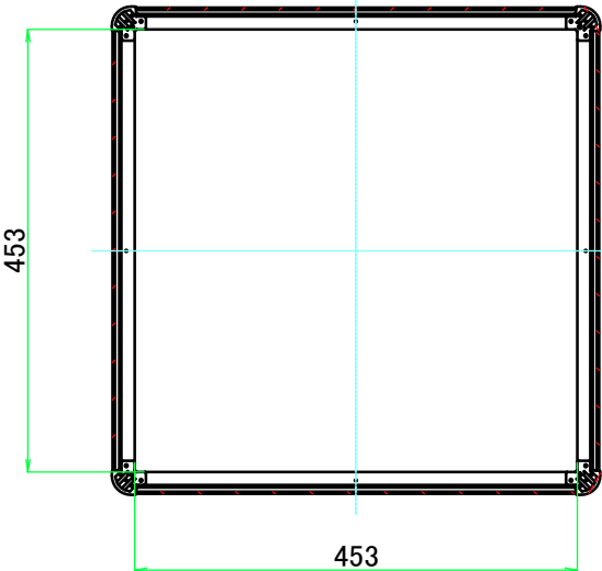
C-C ( 1 : 8.5 )
