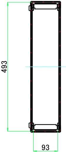
A-A ( 1 : 8.5 )
