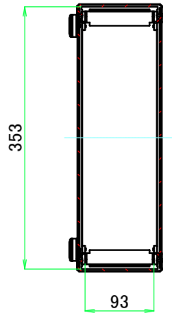
A-A (1:7)
