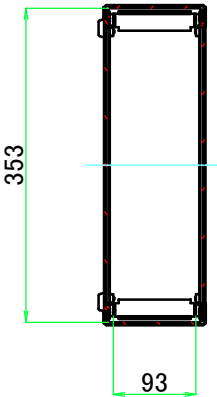
A-A ( 1 : 8.5 )
