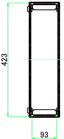
A-A ( 1 : 8.5 )
