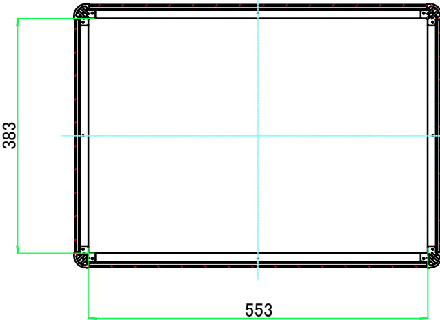
C-C ( 1 : 8.5 )
