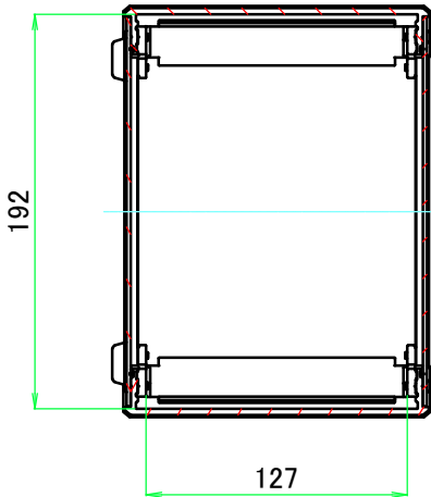
A-A ( 1 : 4 )
