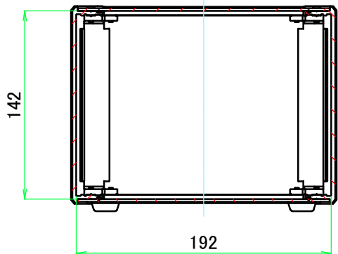
B-B ( 1 : 4 )
