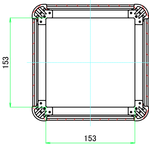
C-C ( 1 : 4 )
