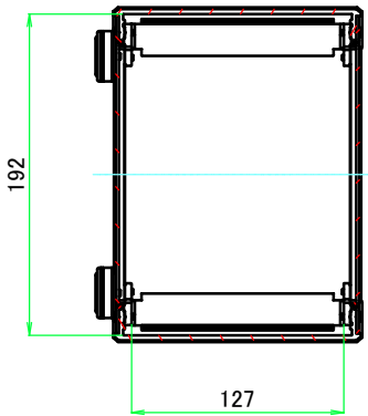
A-A ( 1 : 5 )
