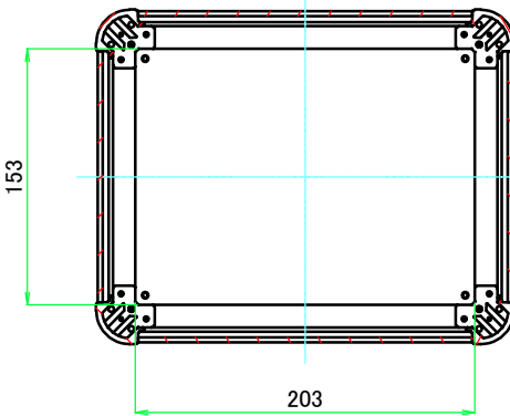
C-C ( 1 : 5 )
