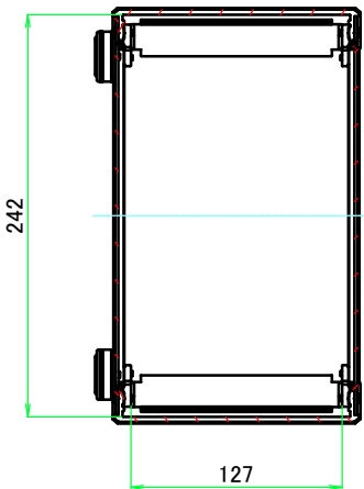
A-A ( 1 : 5 )
