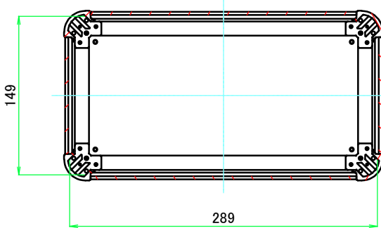
C-C ( 1 : 5 )
