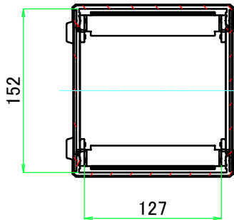
A-A (1:5)
