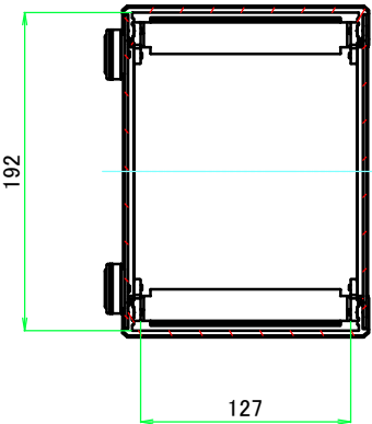
A-A ( 1 : 5 )
