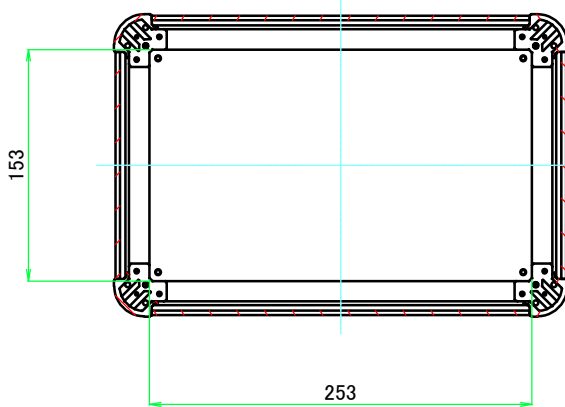
C-C ( 1 : 5 )
