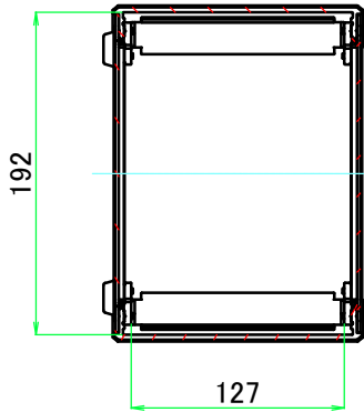
A-A ( 1 : 5 )
