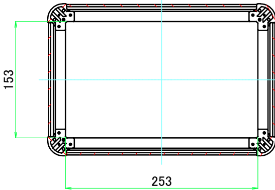
C-C ( 1 : 5 )
