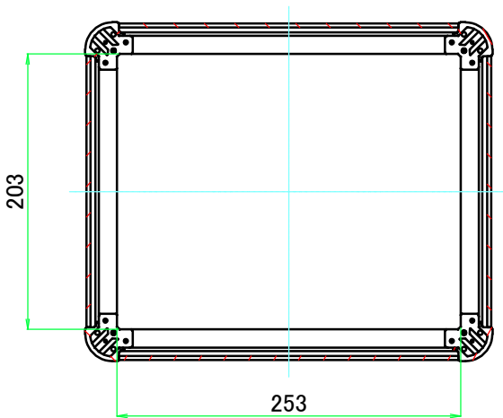
C-C ( 1 : 5 )
