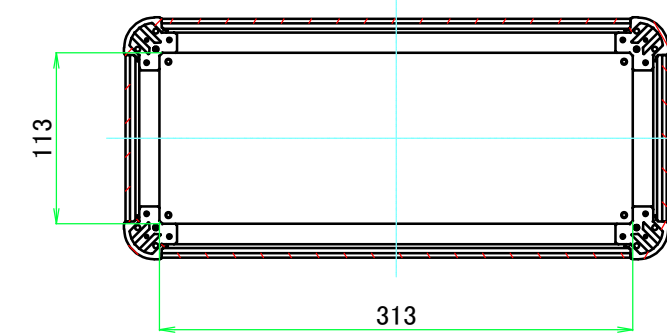
C-C ( 1 : 5 )
