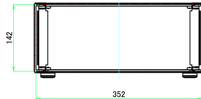
B-B ( 1 : 5 )
