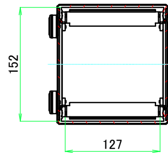
A-A ( 1 : 5 )
