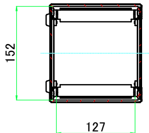
A-A (1:6)
