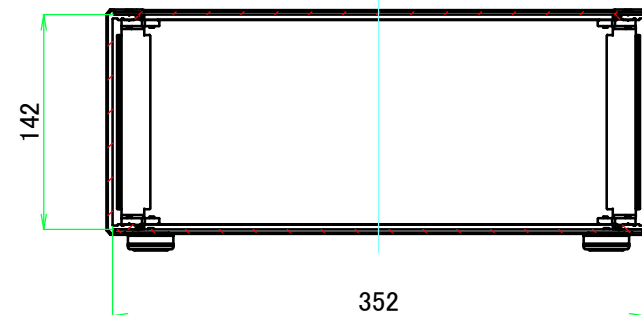
B-B ( 1 : 5 )
