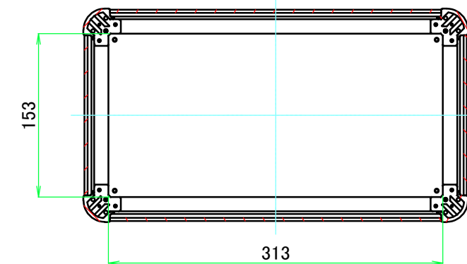
C-C ( 1 : 5 )
