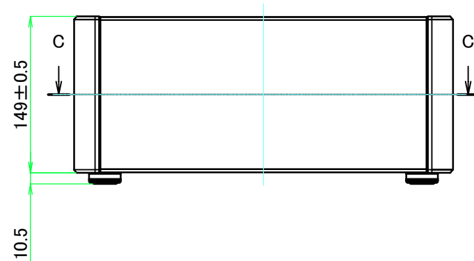
B-B ( 1 : 5 )
