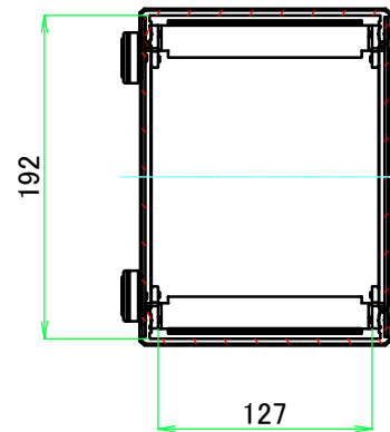
A-A ( 1 : 5 )
