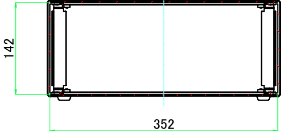
B-B ( 1 : 6 )
