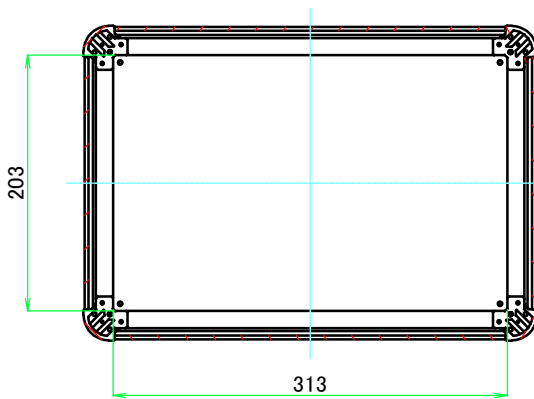
C-C ( 1 : 6 )
