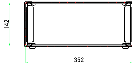
B-B ( 1 : 6 )
