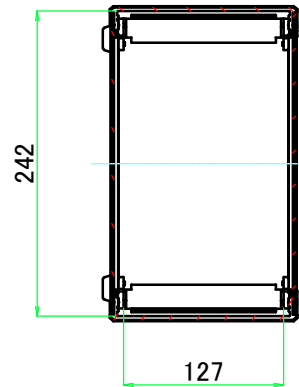
A-A ( 1 : 6 )
