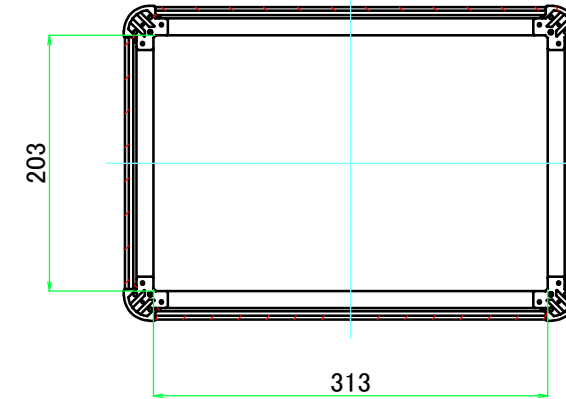
C-C ( 1 : 6 )
