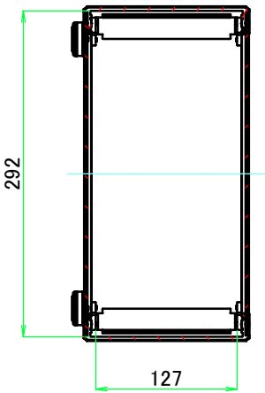
A-A (1:6)
