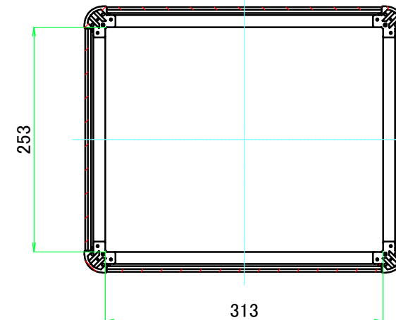
C-C ( 1 : 6 )
