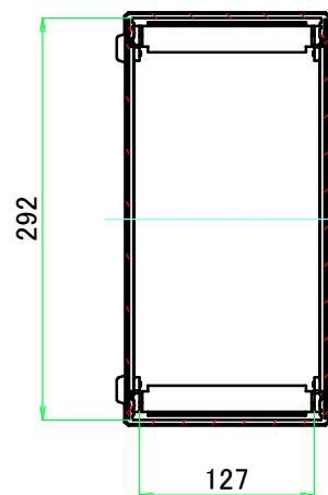
A-A ( 1 : 6 )
