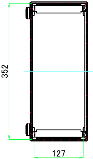
A-A (1:6)
