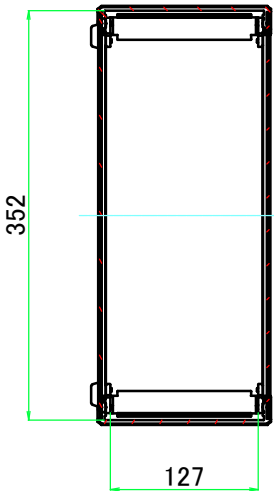
A-A ( 1 : 6.5 )
