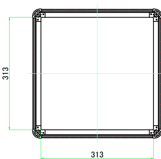
C-C ( 1 : 6.5 )
