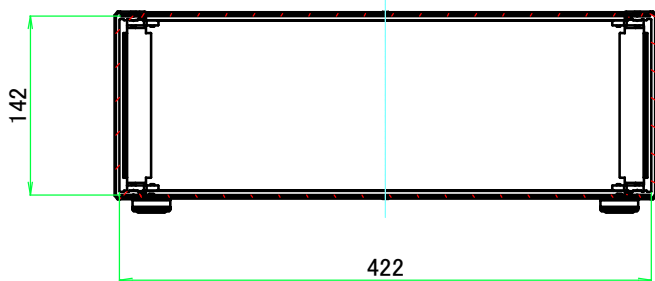
B-B ( 1 : 6 )
