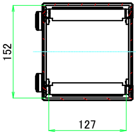
A-A ( 1 : 6 )
