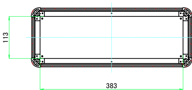
C-C ( 1 : 6 )
