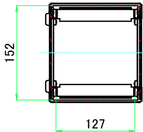
A-A ( 1 : 6 )
