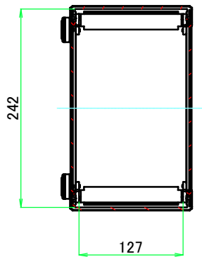
A-A ( 1 : 6.5 )
