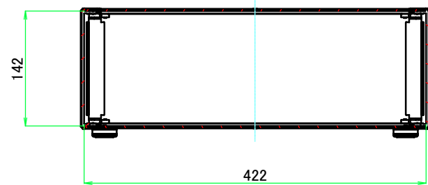
B-B ( 1 : 6.5 )
