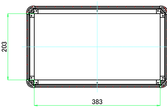
C-C ( 1 : 6 )
