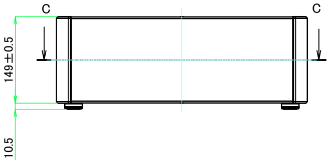
B-B ( 1 : 6.5 )
