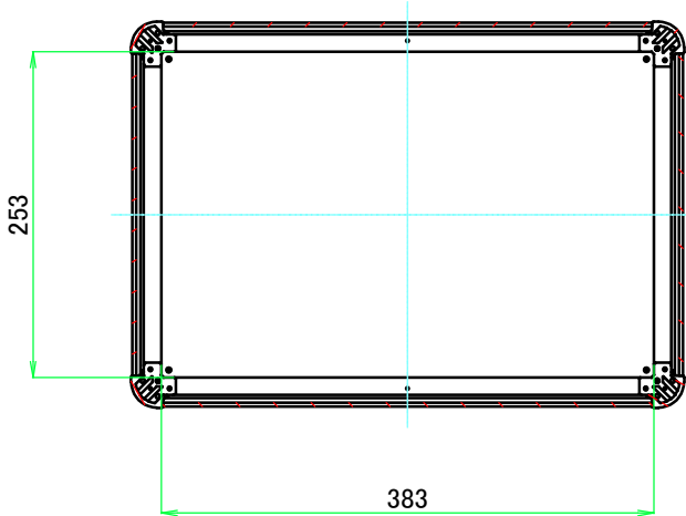
C-C ( 1 : 6.5 )
