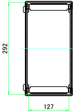
A-A ( 1 : 6 )
