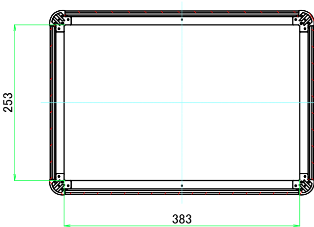
C-C ( 1 : 6 )
