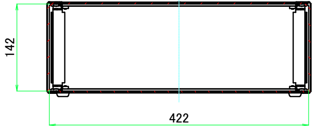
B-B ( 1 : 6 )
