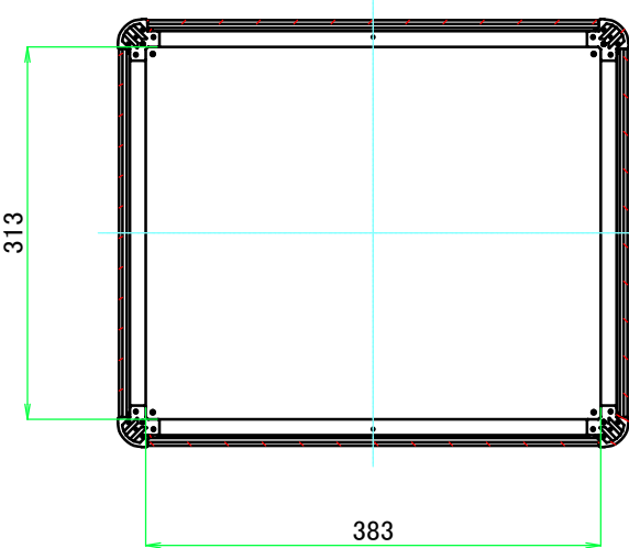
C-C ( 1 : 7 )
