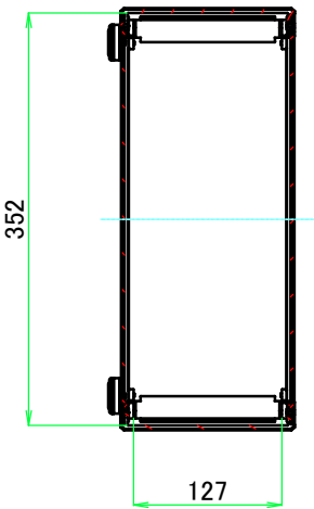
A-A ( 1 : 7 )
