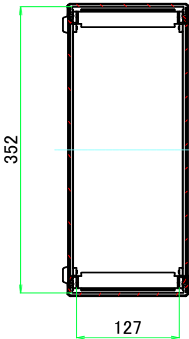
A-A ( 1 : 6.5 )
