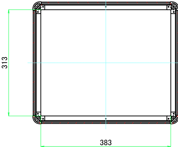
C-C ( 1 : 6.5 )
