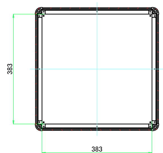
C-C ( 1 : 7.5 )
