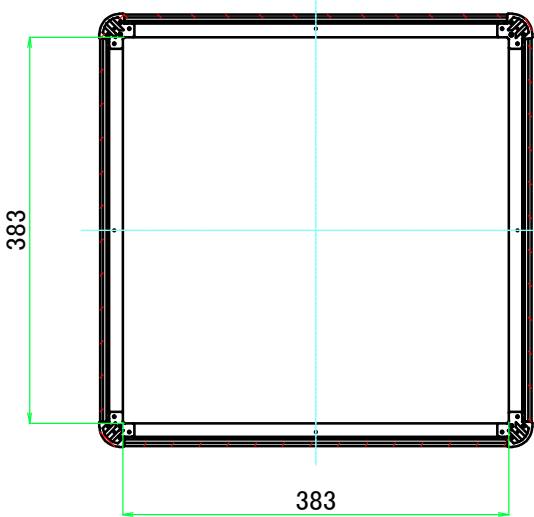
C-C ( 1 : 7.5 )
