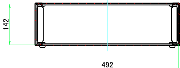
B-B ( 1 : 7.5 )
