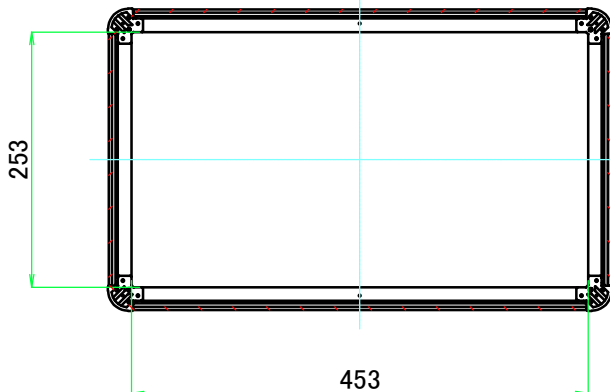
C-C ( 1 : 7.5 )
