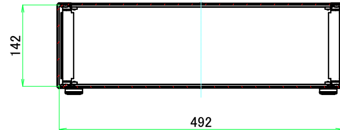
B-B ( 1 : 6.5 )
