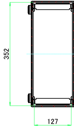
A-A ( 1 : 6.5 )
