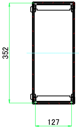
A-A ( 1 : 8 )
