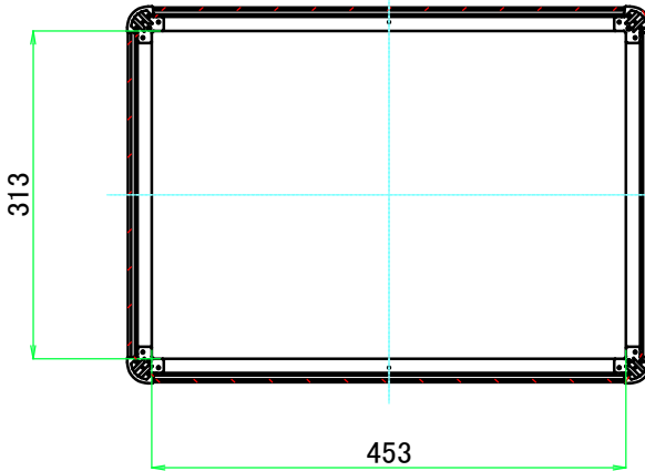
C-C ( 1 : 8 )
