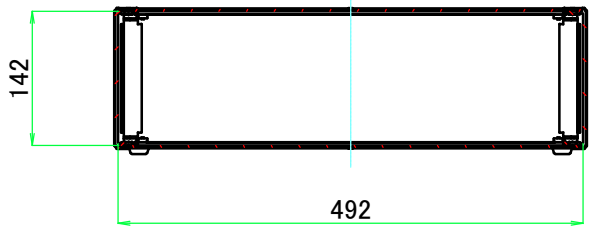
B-B ( 1 : 8 )
