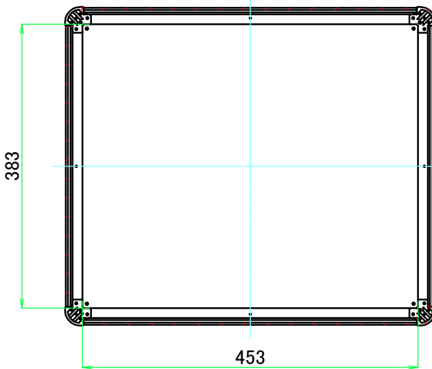
C-C ( 1 : 7 )
