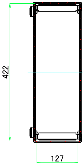
A-A ( 1 : 7 )
