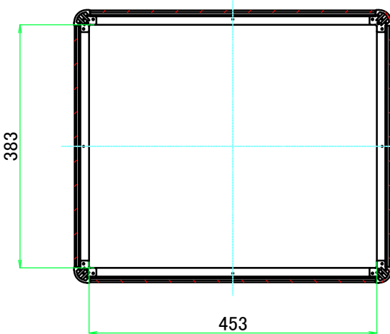
C-C ( 1 : 8.5 )
