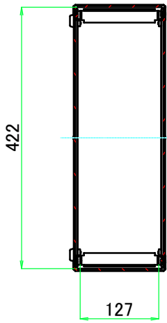
A-A ( 1 : 8.5 )
