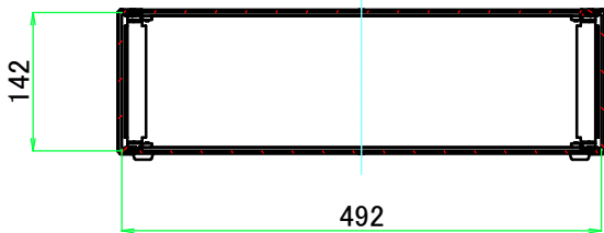
B-B ( 1 : 8.5 )
