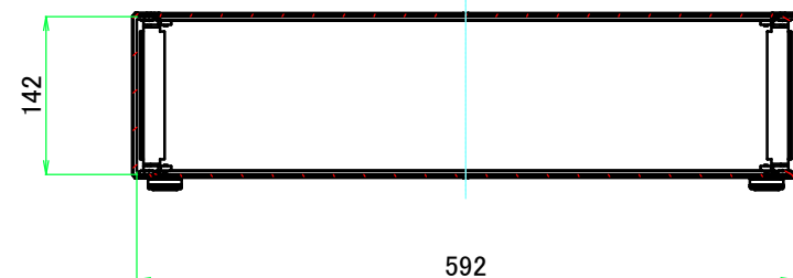
B-B ( 1 : 7.5 )
