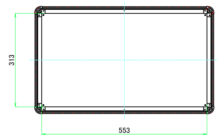
C-C ( 1 : 7.5 )
