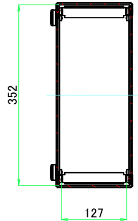
A-A ( 1 : 7.5 )
