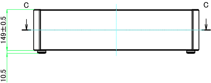
B-B ( 1 : 8 )
