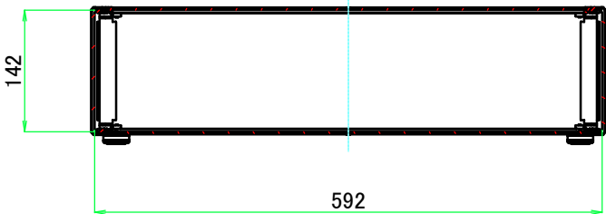
B-B ( 1 : 8 )
