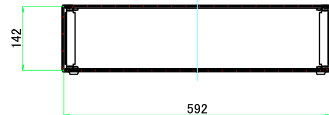
B-B ( 1 : 8.5 )
