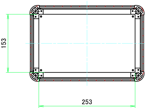
C-C ( 1 : 5 )
