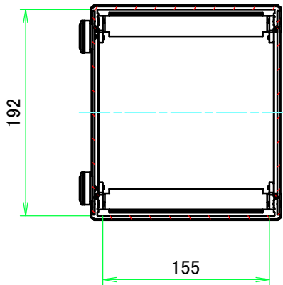
B-B ( 1 : 5 )
