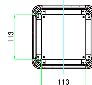
C-C ( 1 : 5.5 )
