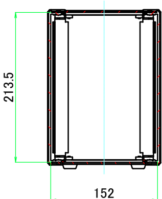
B-B ( 1 : 5.5 )
