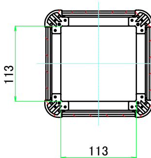
C-C ( 1 : 5.5 )
