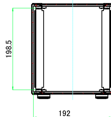
B-B ( 1 : 5.5 )
