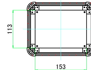
C-C ( 1 : 5.5 )
