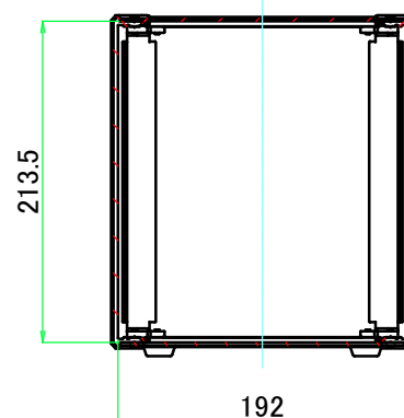
B-B ( 1 : 5.5 )
